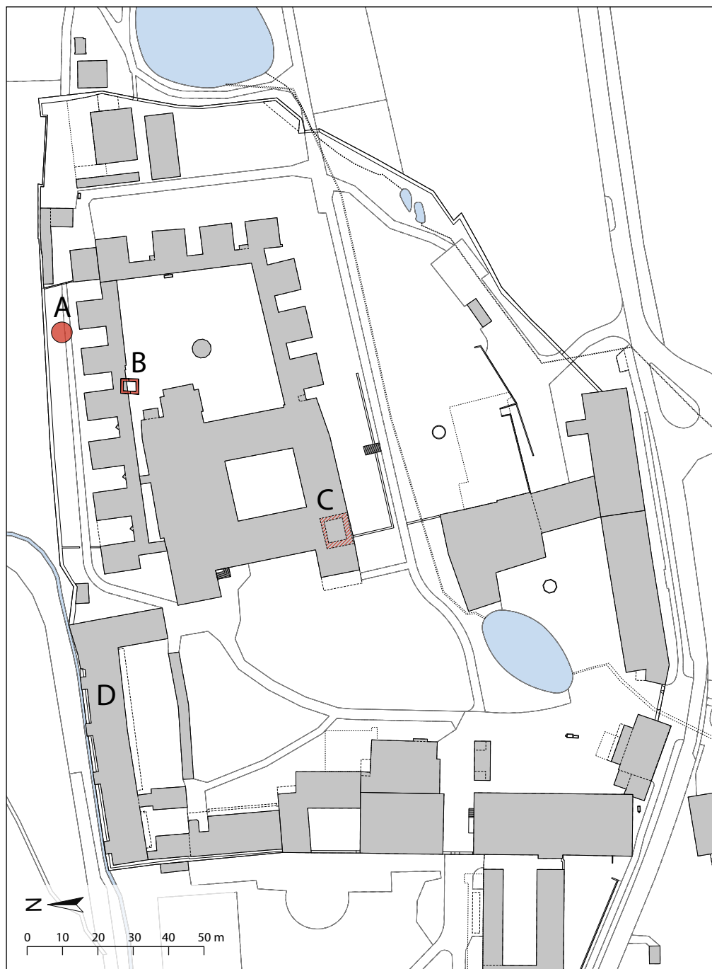
7: Warth-Weiningen TG, Kartause Ittingen. Übersichtsplan mit vorkartausezeitlichen Befunden; A) Kalkbrennofen, B) rechteckiger Gebäudegrundriss, C) vermuteter, archäologisch nicht nachgewiesener «Wohnturm», D) ungefähre Lage des «Megalithmauerwerks».
