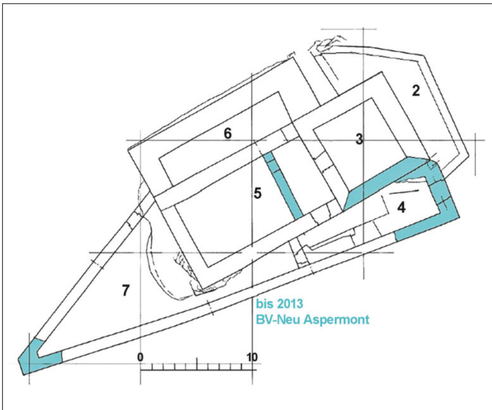
12: Grundriss Burg Neu-Aspermont. Blau markiert die Notsicherungen und Konservierungsarbeiten am Gemäuer 1999 bis 2013.
