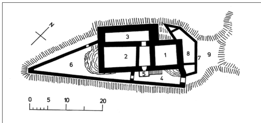
2: Grundriss Burg Neu-Aspermont. 1: Wohnturm, 2: Palas, 3: Anbau, 4: Zwinger – Hof, 5: Podest und Treppe, 6: Hof, 7: Futtermauer, 8: Berme, 9: Halsgraben.
