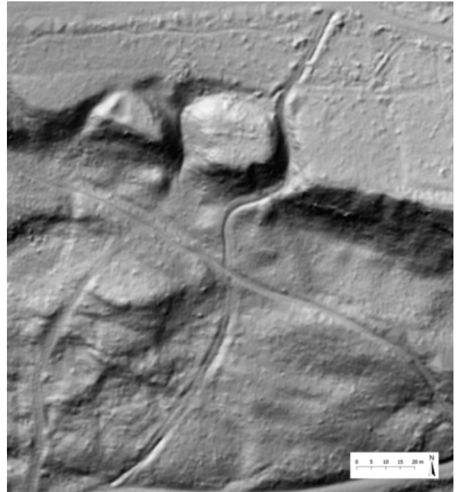
2: Uesslingen-Buch TG, Burgstelle Töbeli. Reliefkarte (LIDAR) mit den beiden Plateaus, Gräben sowie Wegstrukturen.
