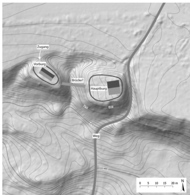
3: Uesslingen-Buch TG, Burgstelle Töbeli. Topografischer Plan und Rekonstruktionsvorschlag der Burgstelle.
